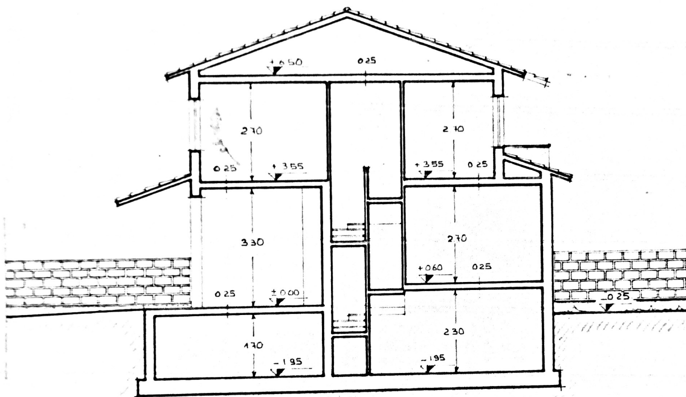
SEZIONE Z-Z
